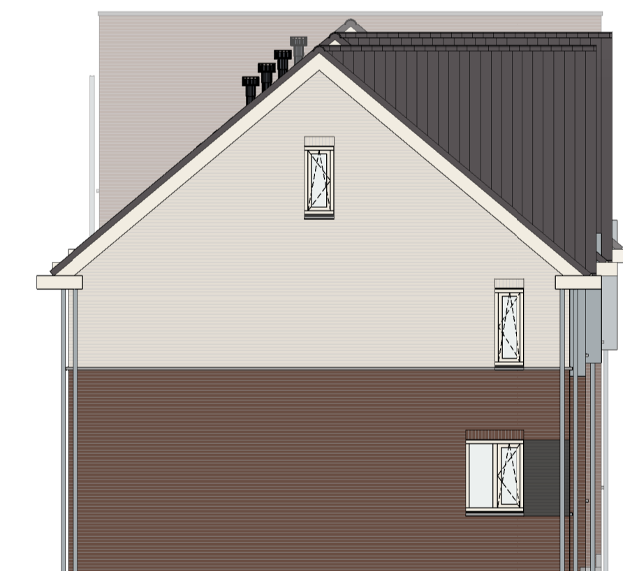
linkergevel 1 : 100
